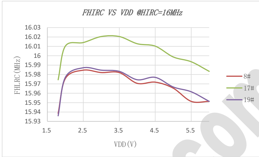
HIRC 频率 VS 电源电压/温度
