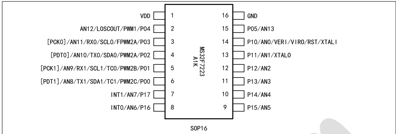
图 1-2 MS32F7223A1K
