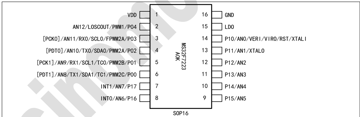
图 1-1 MS32F7223A0K
