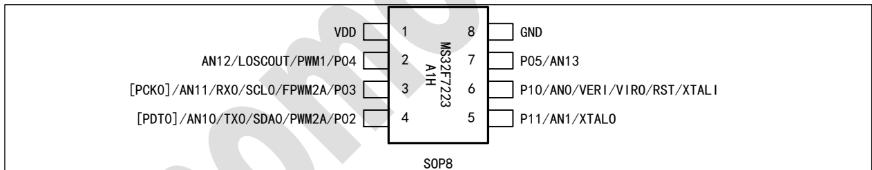
图 1-4 MS32F7223A1H
