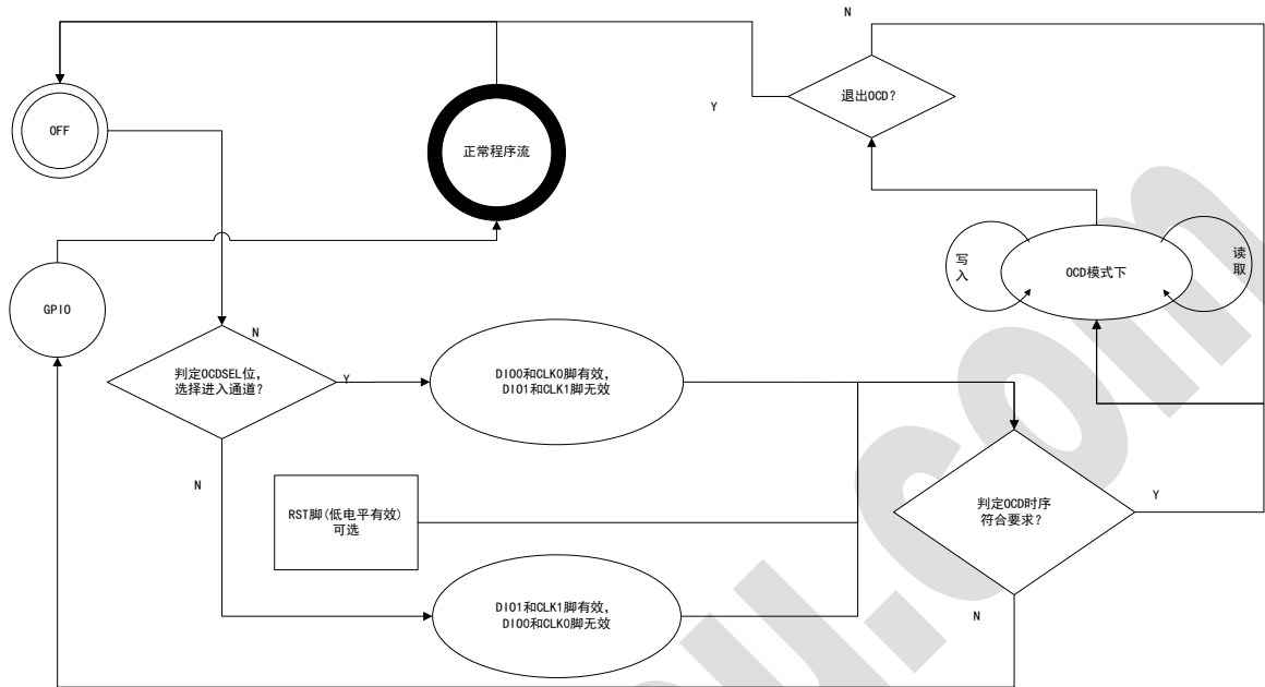
OCD状态机示意图
