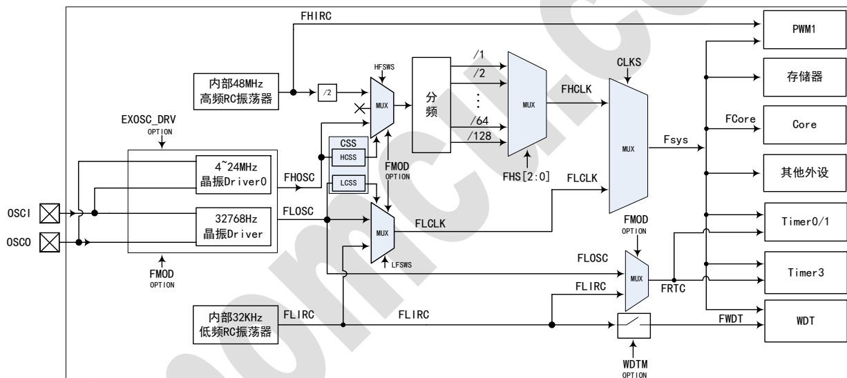
系统时钟示意图
